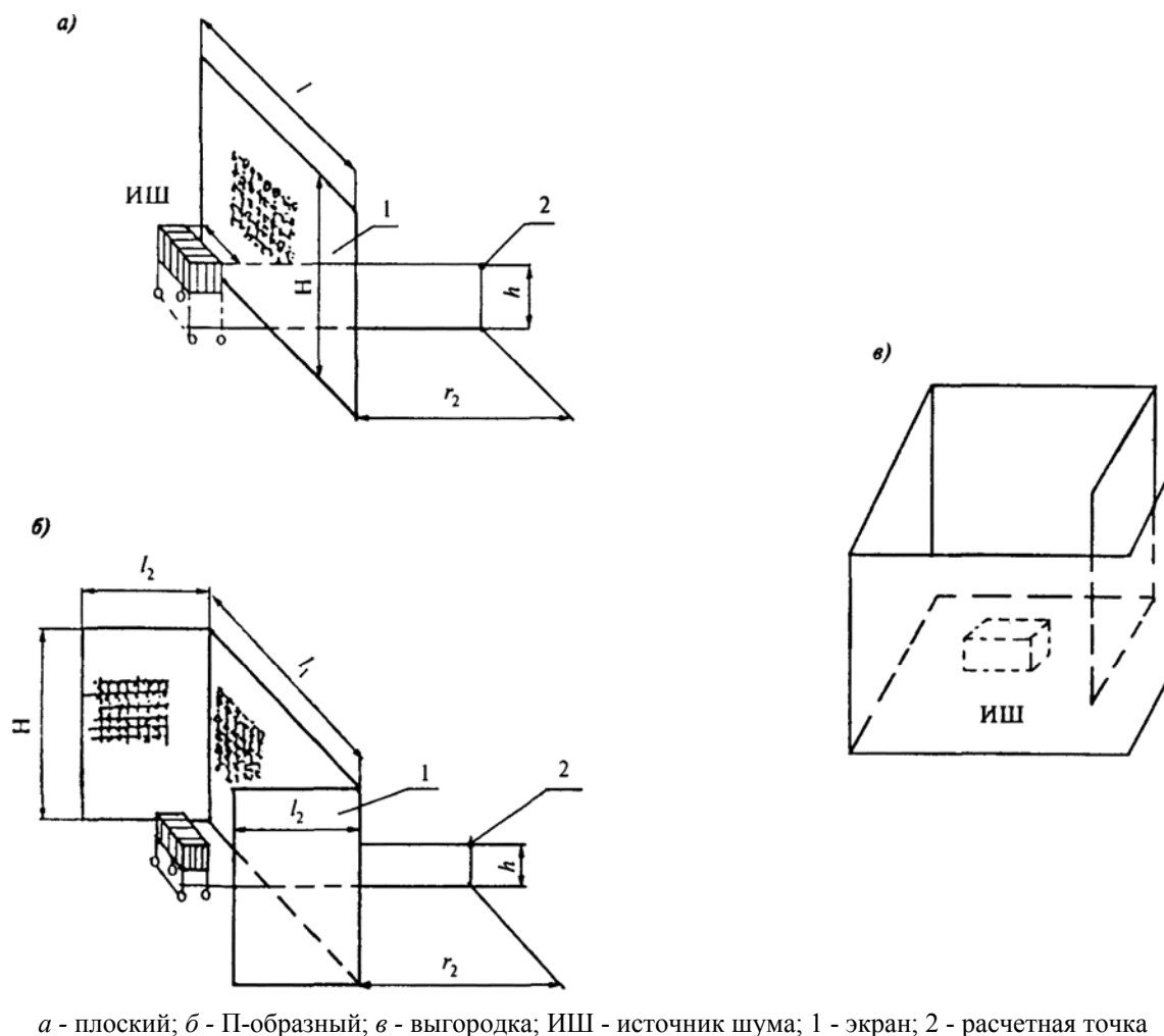
Рисунок 5 - Формы акустических экранов
